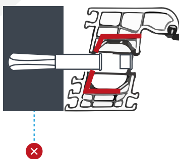
FÖNSTERKARMENS TVÄRBÖJNING
