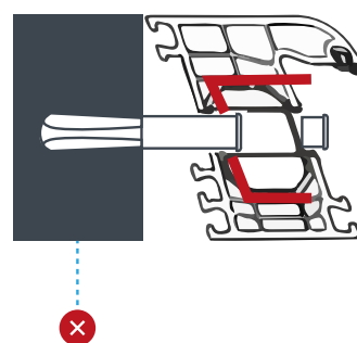
FÖNSTERKARMENS TVÄRBÖJNING
